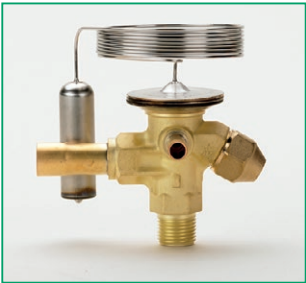
TEV - Termosztatikus expanziós szelep
